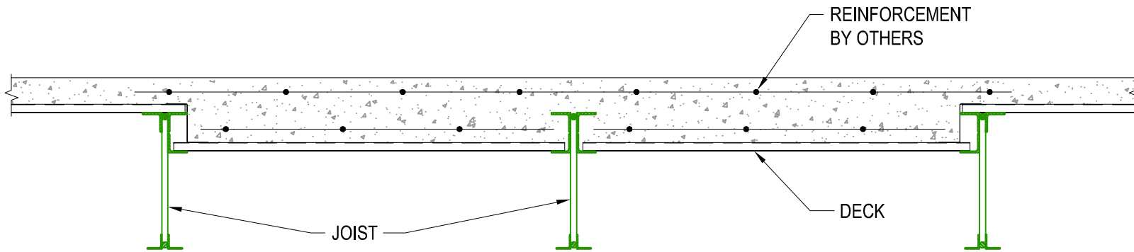
SECTION A-A
